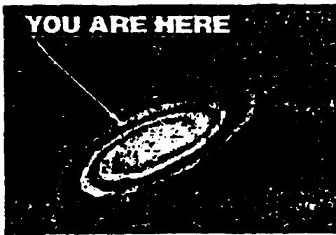
٣ - موقعنا في مجرة درب التبانة
